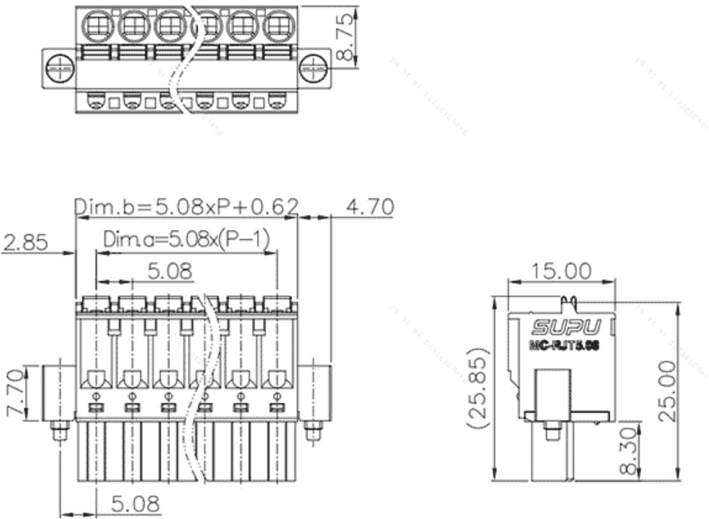
产品尺寸图
