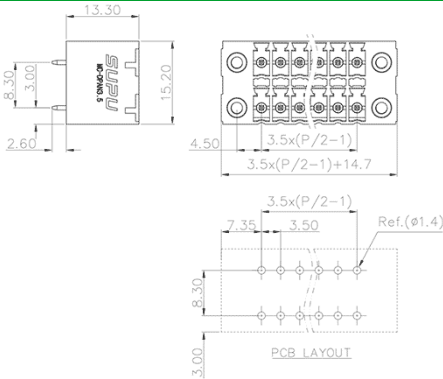
产品尺寸图
