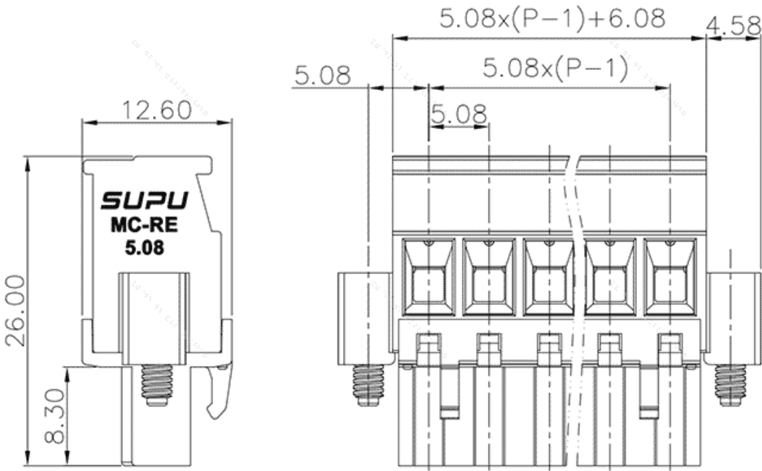
产品尺寸图
