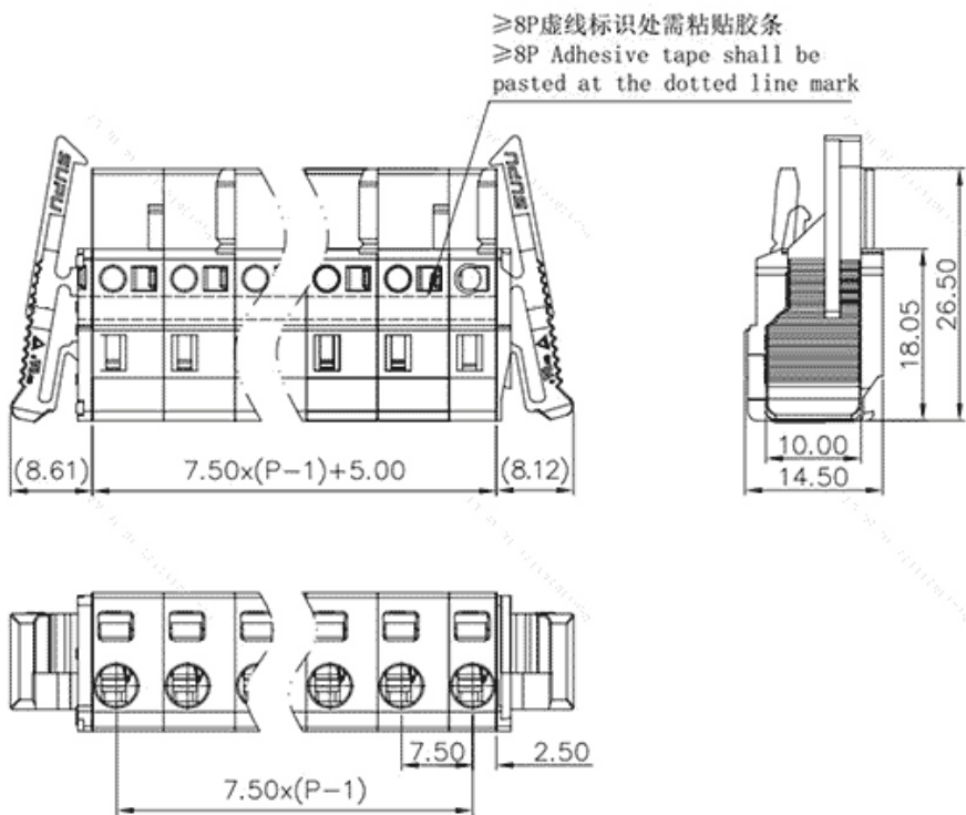
产品尺寸图
