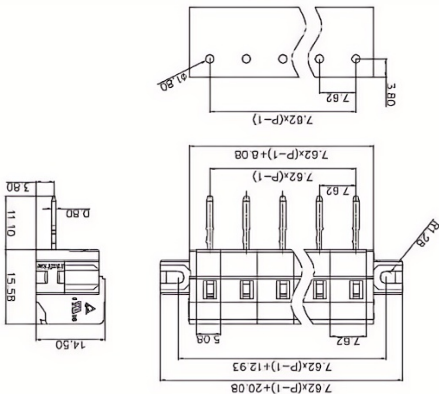
产品尺寸图
