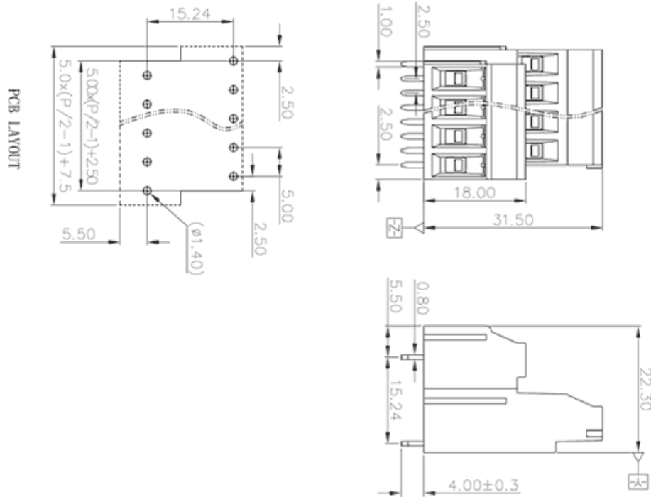
产品尺寸图
