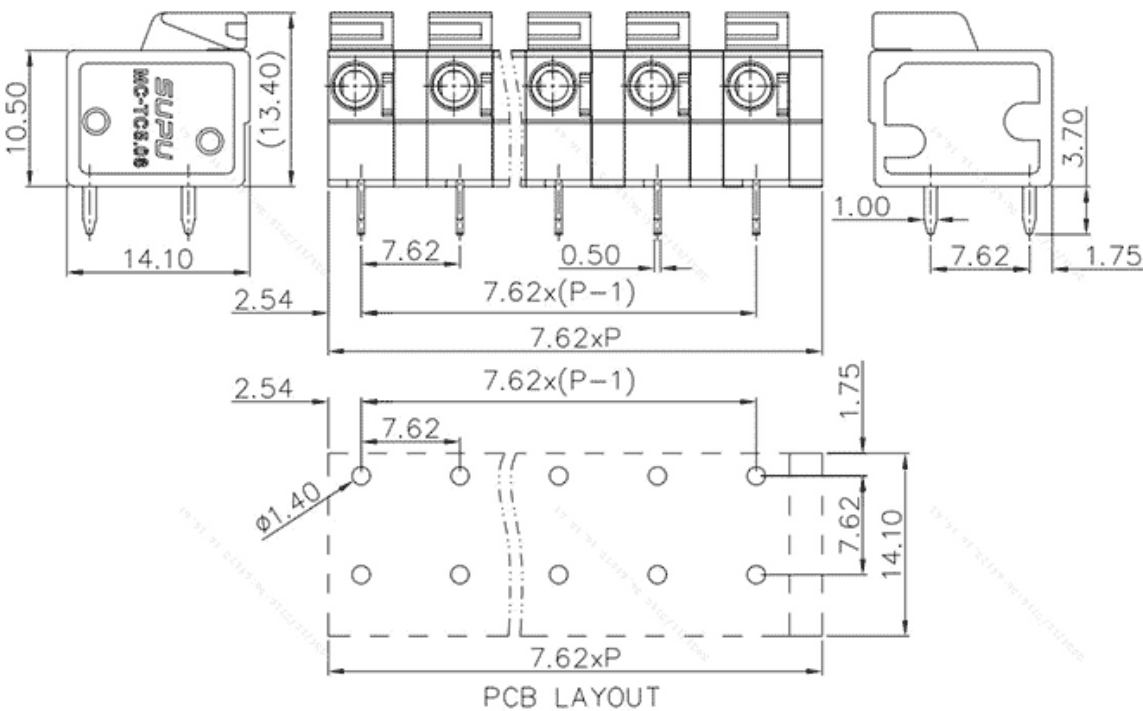
产品尺寸图
