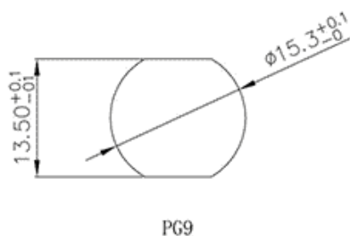
安装尺寸 Installation dimension
