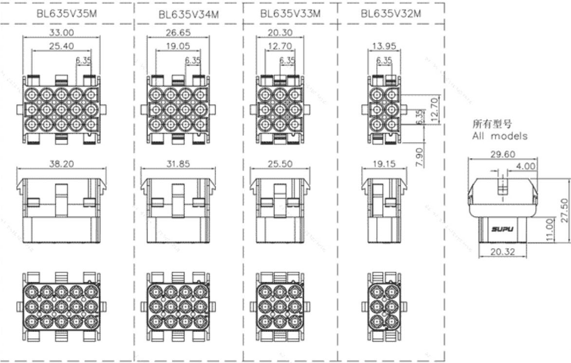
产品尺寸图
