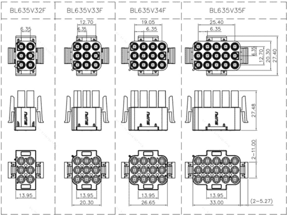
产品尺寸图
