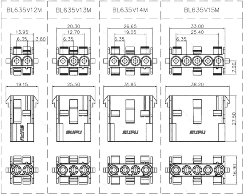
产品尺寸图
