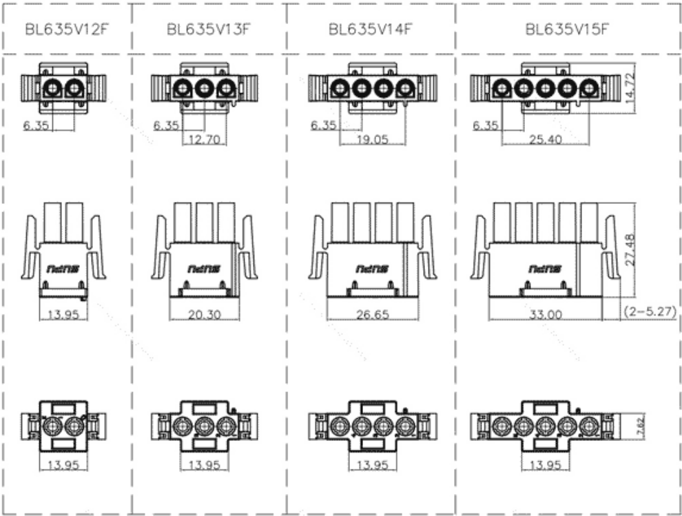
产品尺寸图
