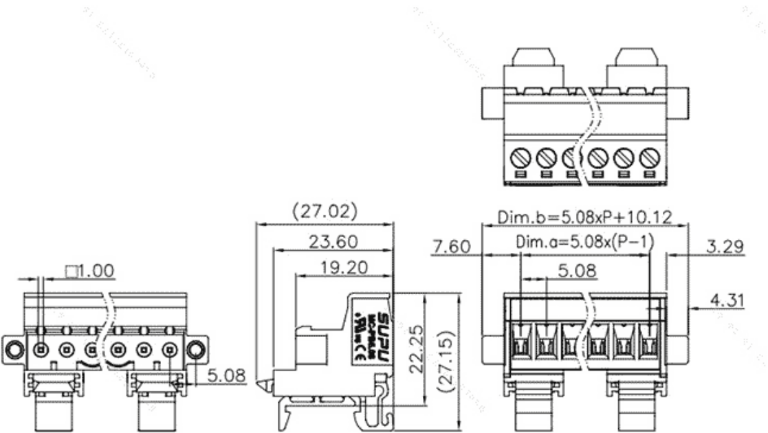
产品尺寸图
