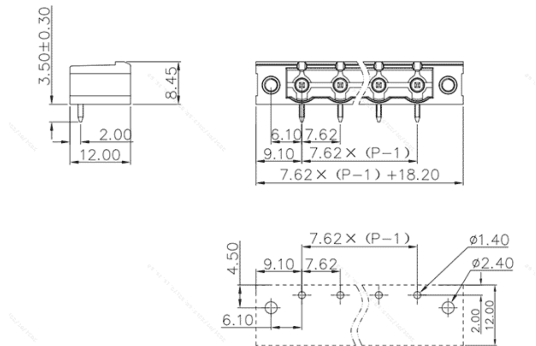
产品尺寸图
