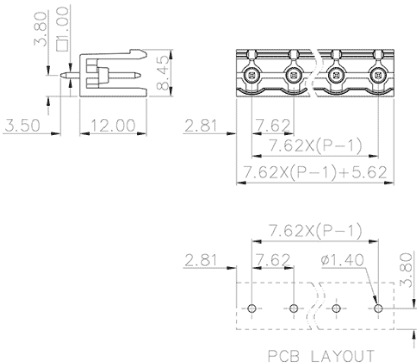
产品尺寸图
