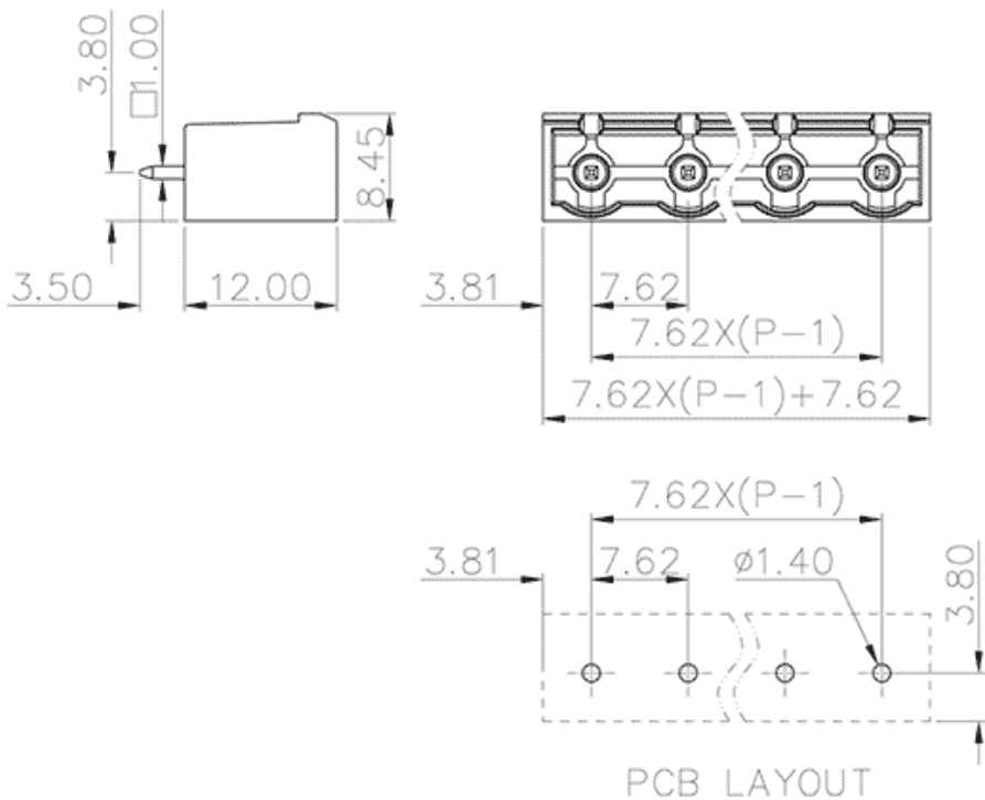
产品尺寸图
