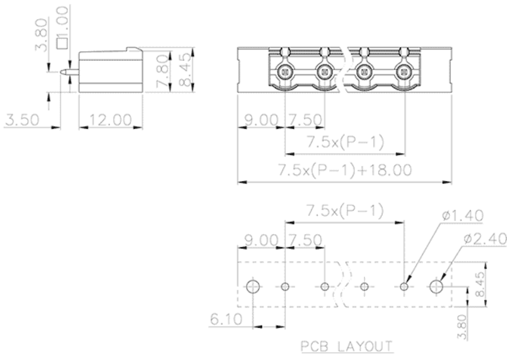
产品尺寸图
