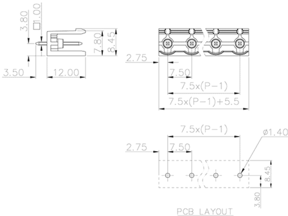
产品尺寸图
