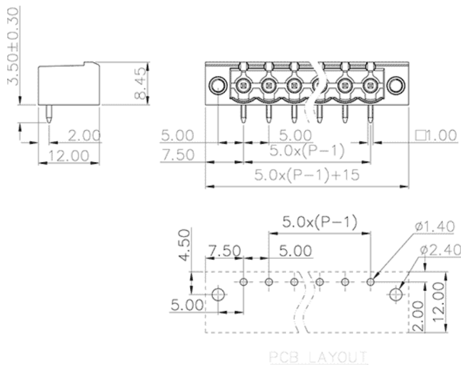
产品尺寸图
