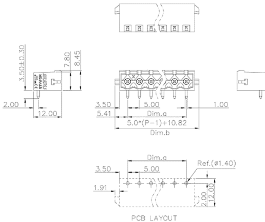
产品尺寸图
