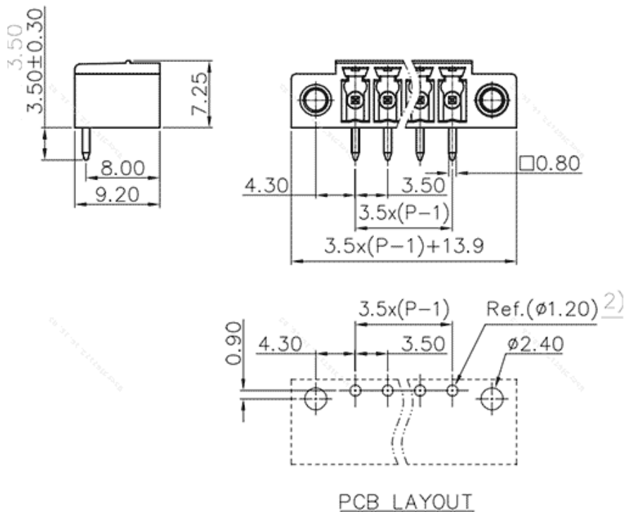
产品尺寸图
