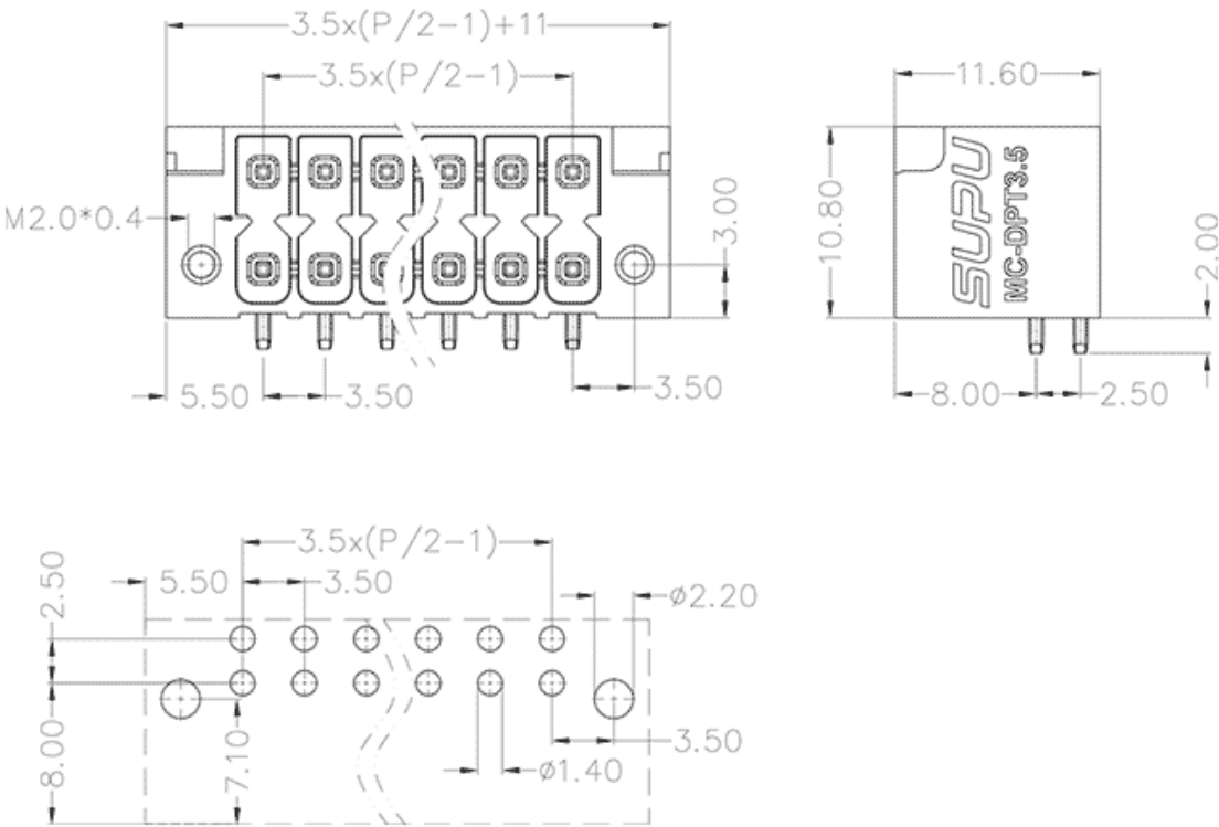
产品尺寸图
