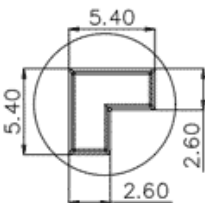
5:1 L形导光柱
