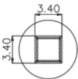
5:1 方形导光柱
