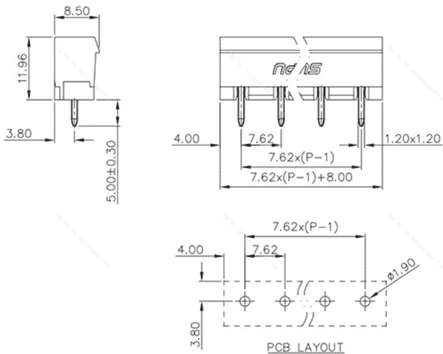
产品尺寸图
