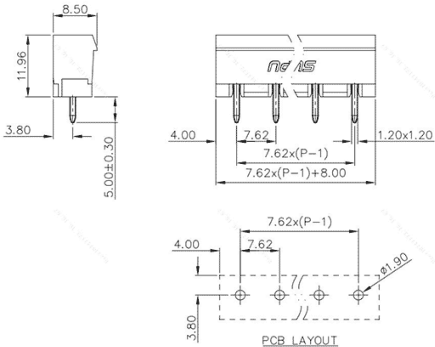
产品尺寸图
