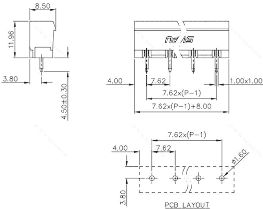
产品尺寸图
