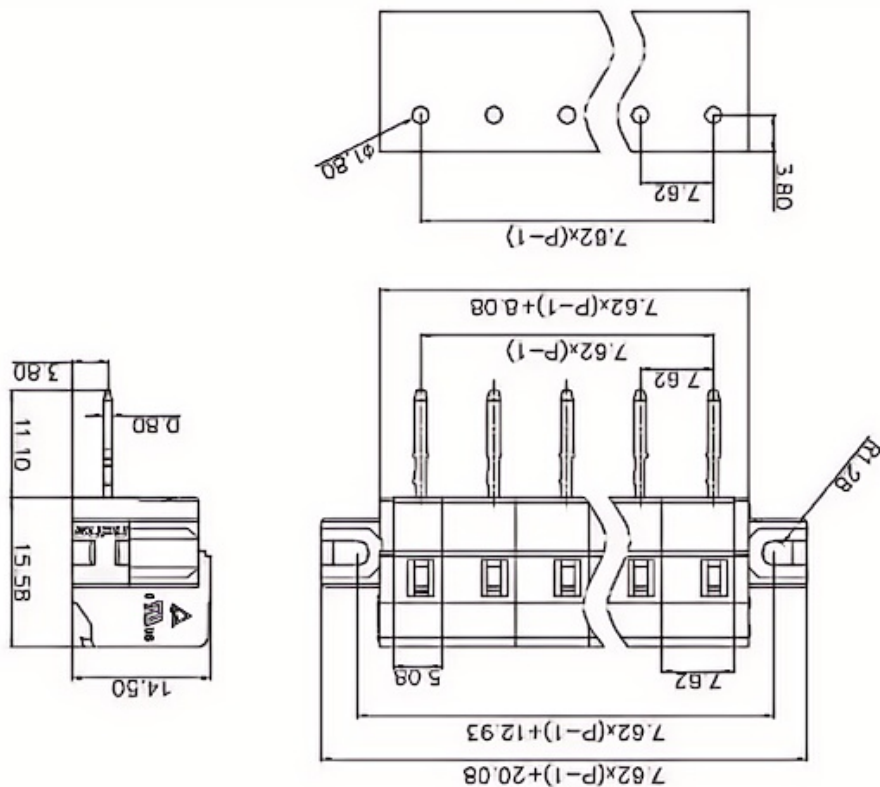
产品尺寸图
