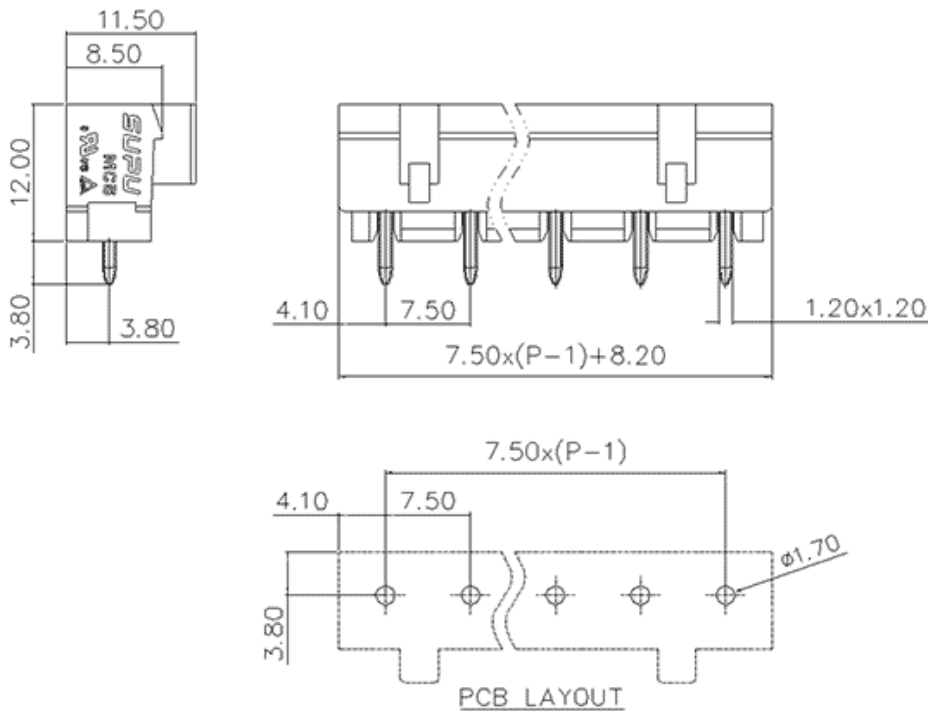
产品尺寸图
